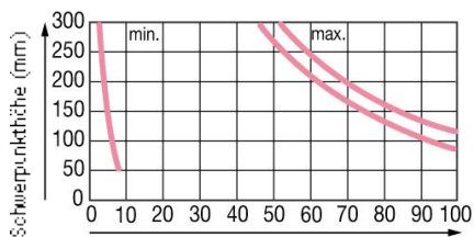
Kameraplattform Counterbalance
