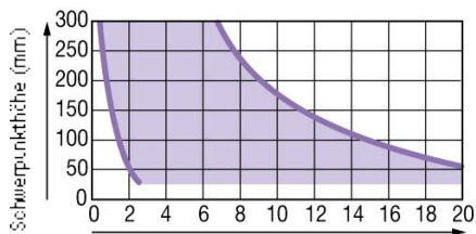
Kameraplattform Counterbalance
