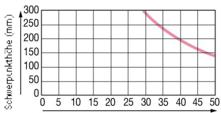
Kameraplattform Counterbalance
